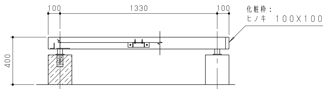
正面図 S = 1/20
