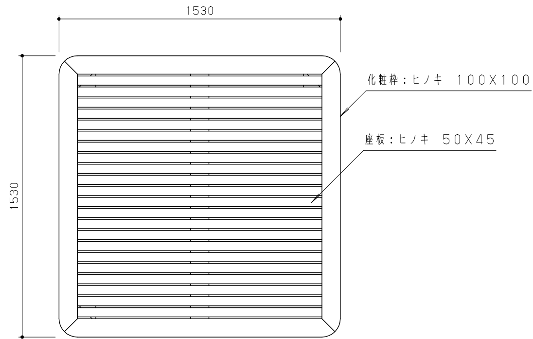
平面図 S = 1/20
