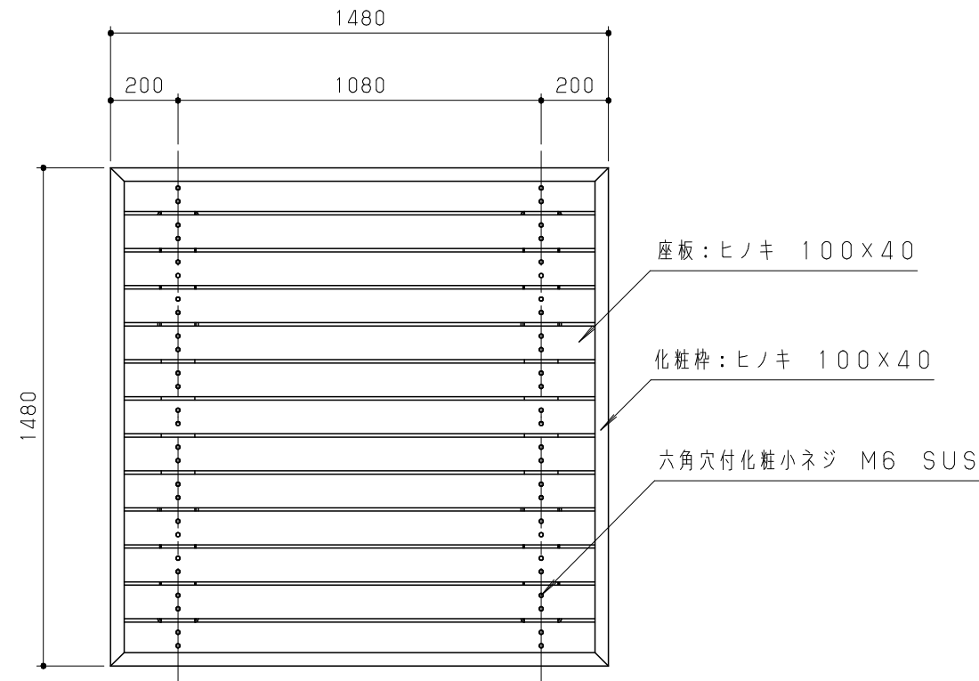
平面図 S=1/20
