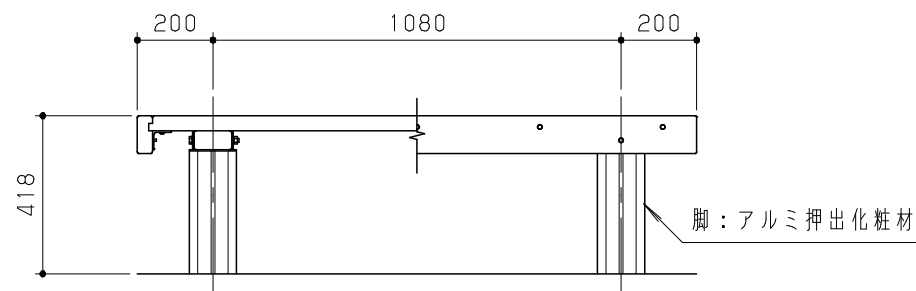
正面図 S=1/20
