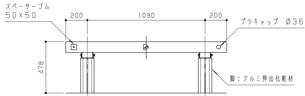
正面図 S=1/20
