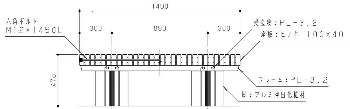
側面図 S=1/20
