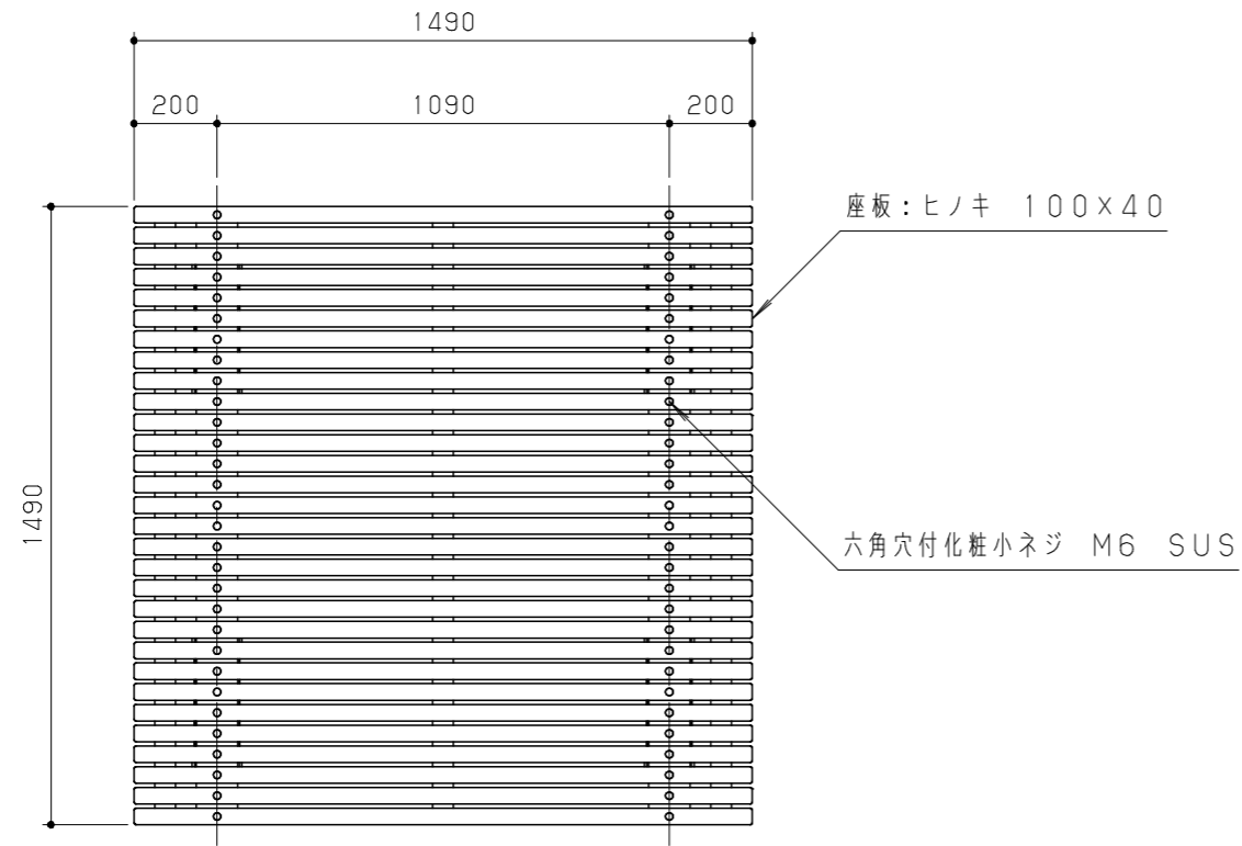
平面図 S=1/20
