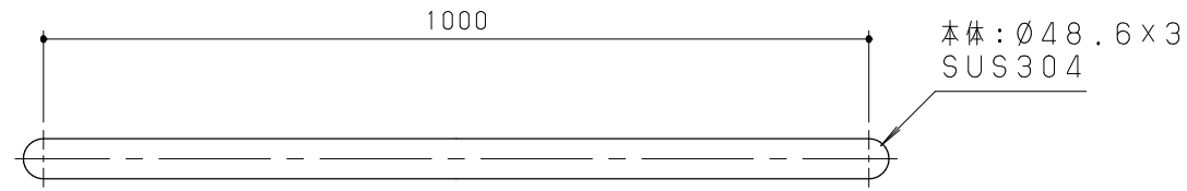
平面図 S = 1 / 10
