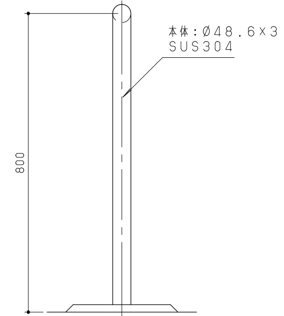
側面図 S = 1 / 10
