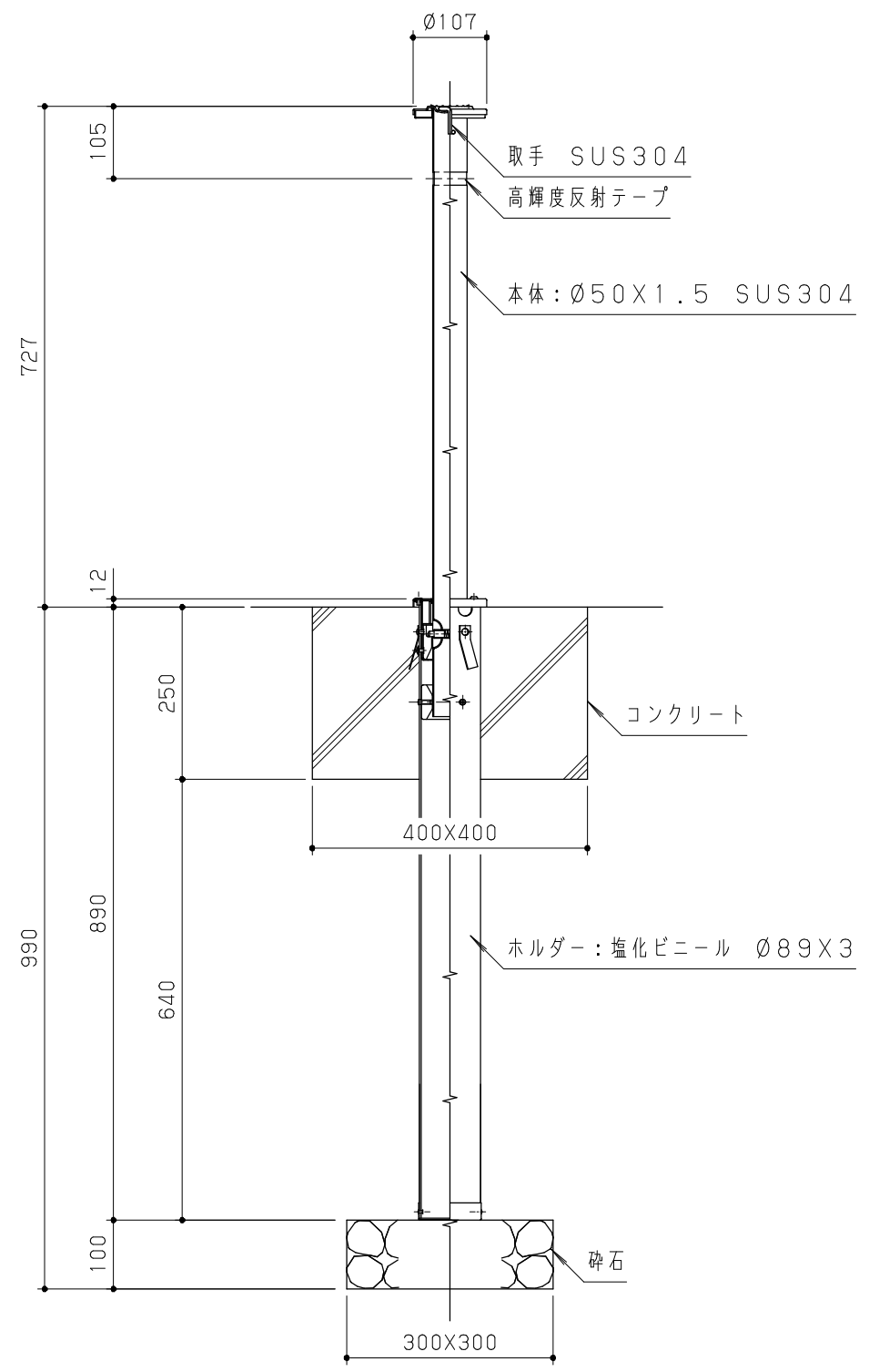
立断面図 S = 1 / 10
