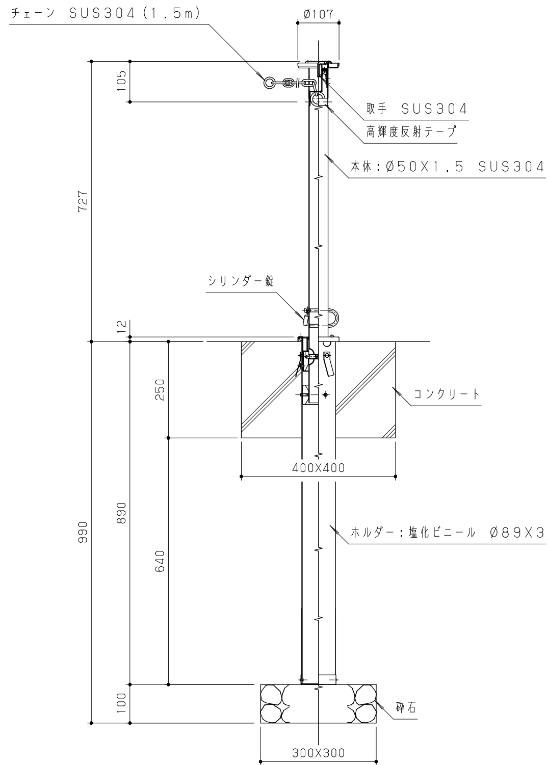
立断面図 S = 1 / 10
