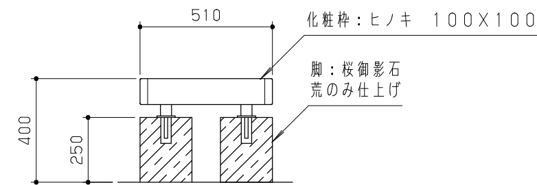
側面図 S=1/20
