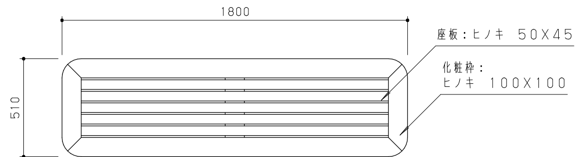
平面図 S=1/20
