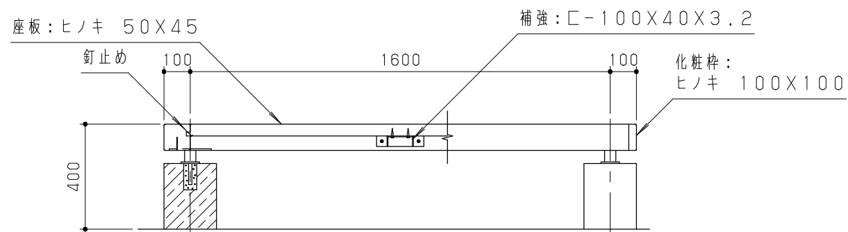
正面図 S=1/20
