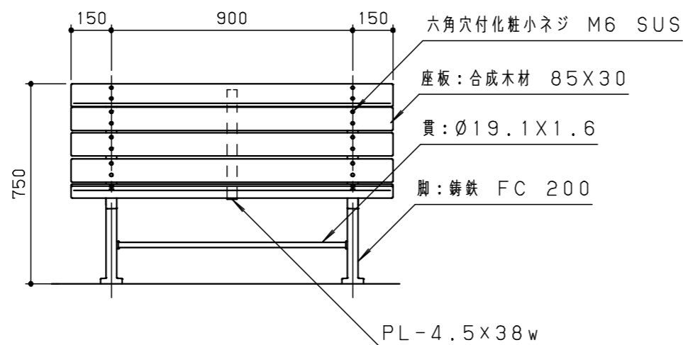
正面図 S = 1/20
