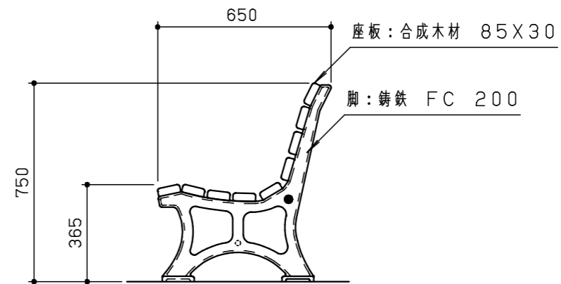
側面図 S = 1/20
