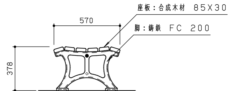
側面図 S=1/20
