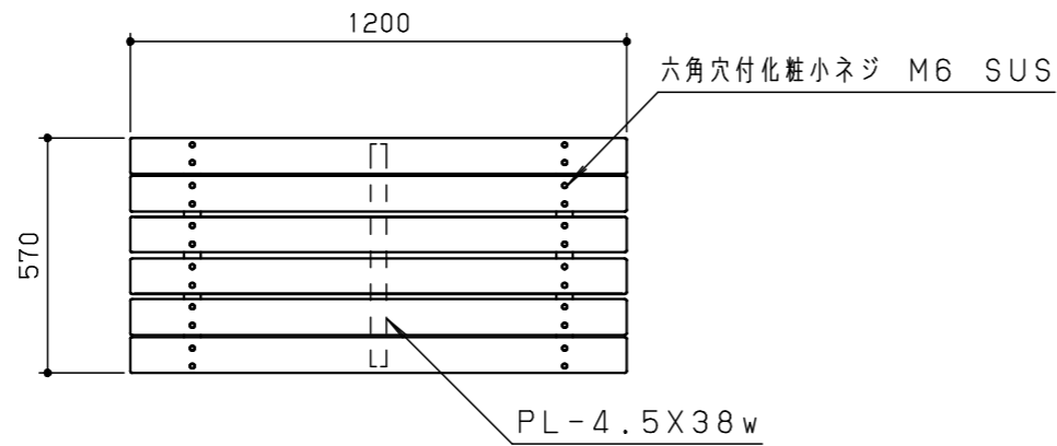
平面図 S=1/20
