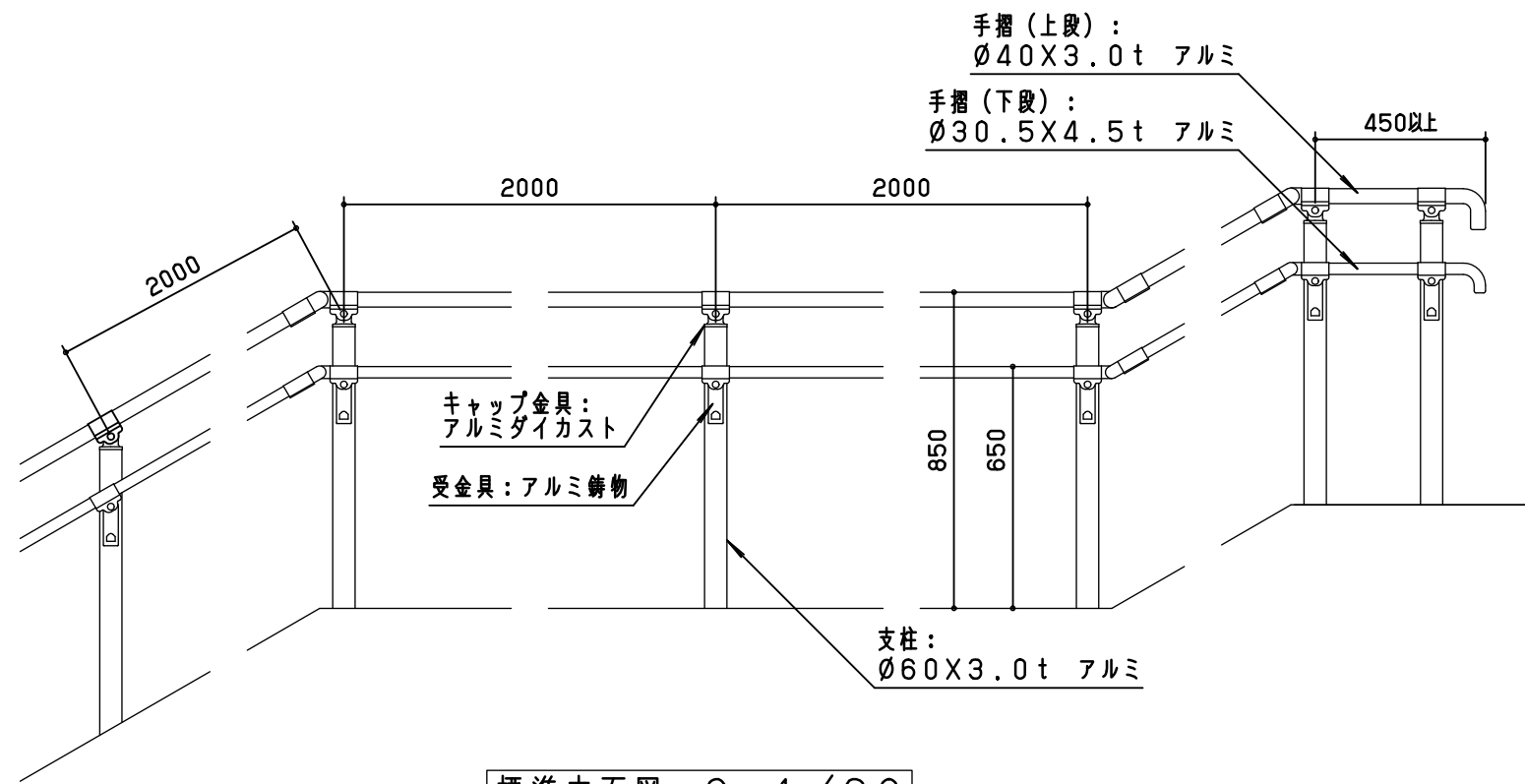
標準立面図 S=1/20
