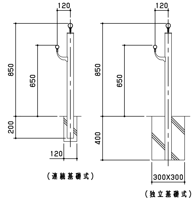
標準断面図 S=1/20
