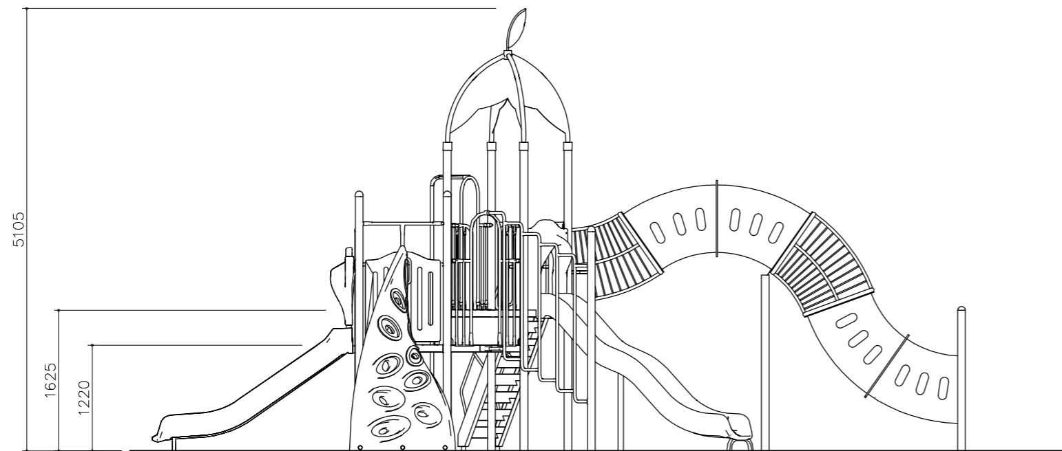
立面図 S=1/60
