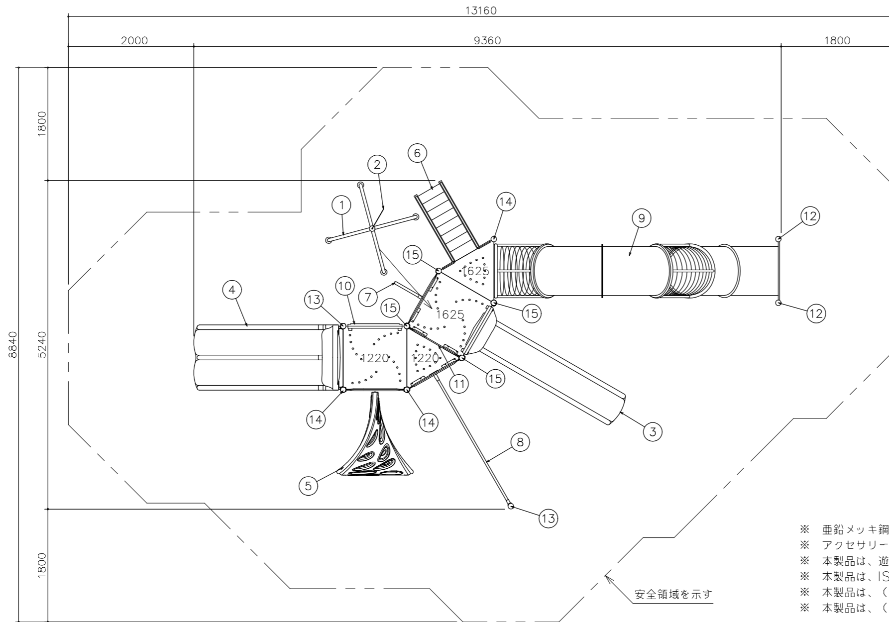
平面図 S=1/60
