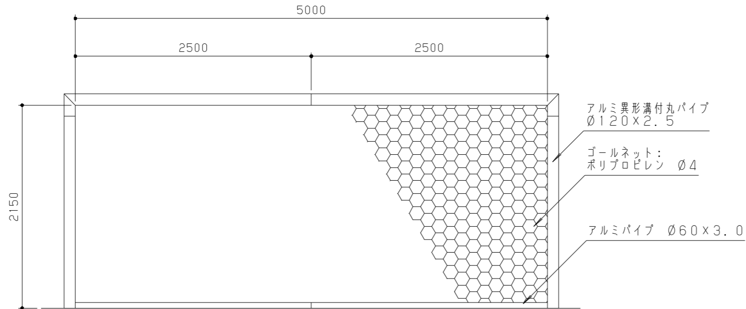
正面図 S = 1 / 40
