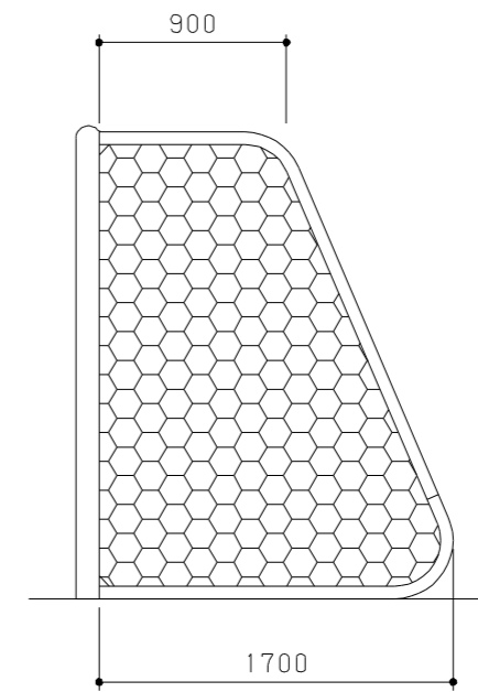
側面図 S = 1 / 40
