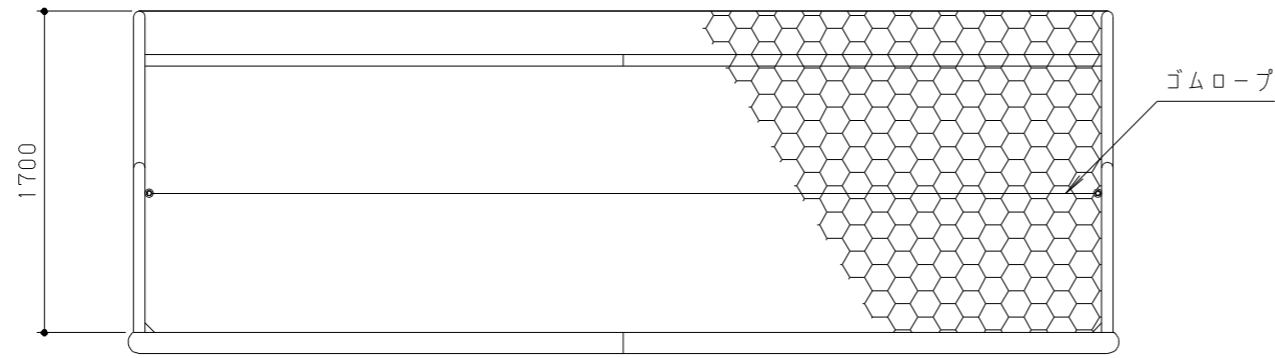
平面図 S = 1 / 40
