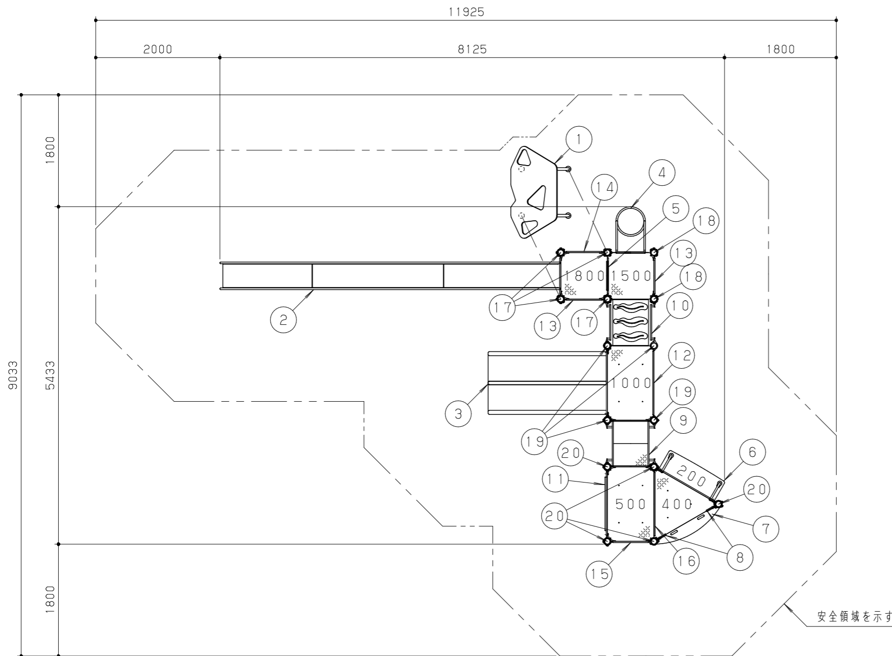
平面図 S = 1 / 60
