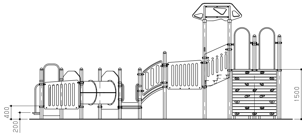
C 視立面図 S = 1 / 60
