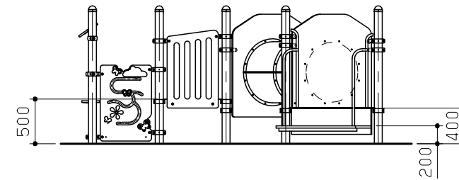
B 視立面図 S = 1 / 60
