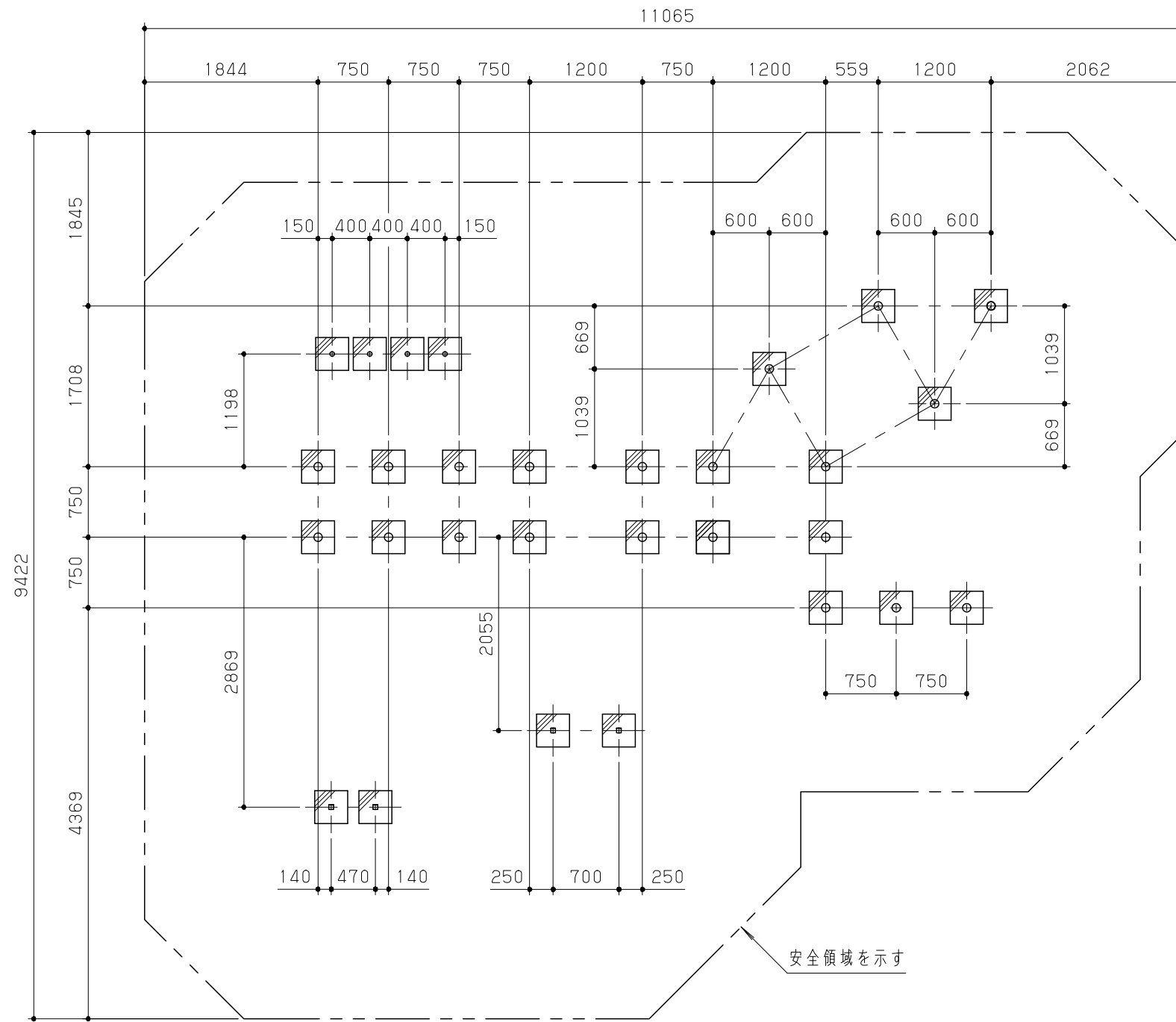
基礎伏図 S = 1 / 60
