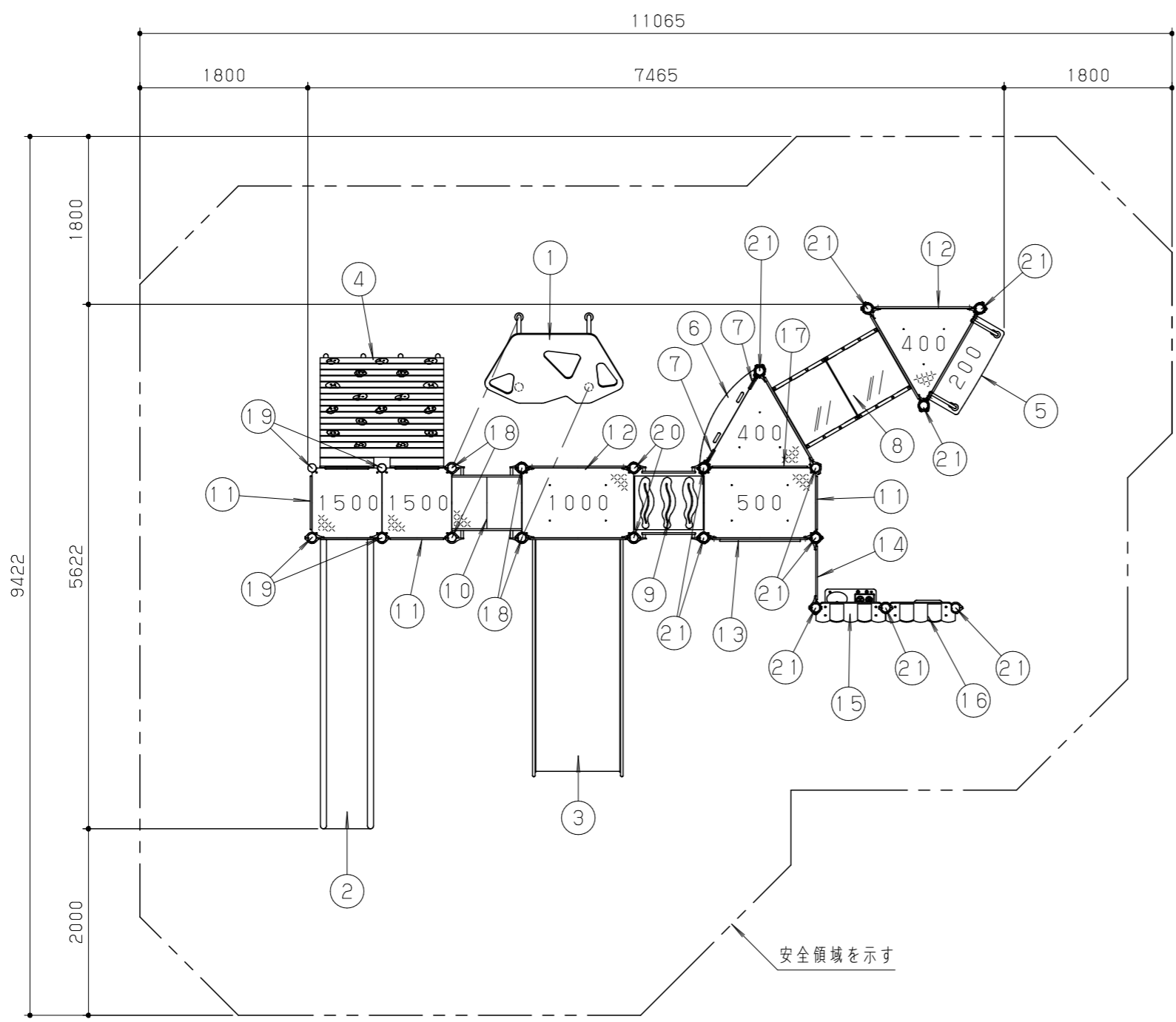
平面図 S=1/60
